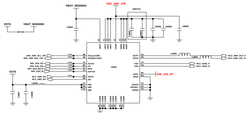
RCV AMP
