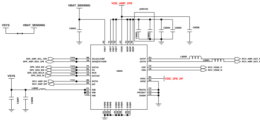
RCV AMP
