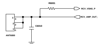
RCV CONTACT
