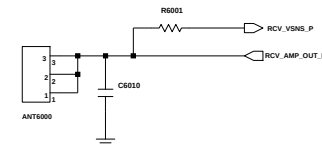
RCV CONTACT
