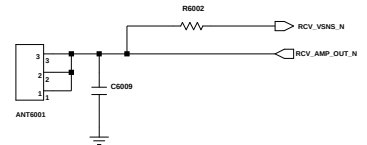
RCV CONTACT
